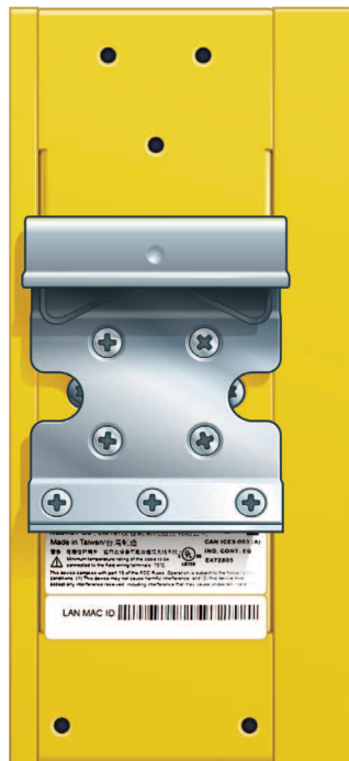
Fig. 4: NoriGate V2 - DIN rail-mounted
